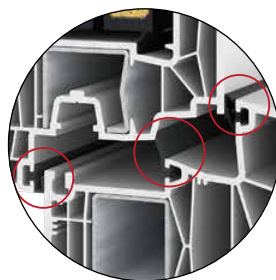
Systém středového těsnění
