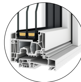
Nízký podlahový práh
