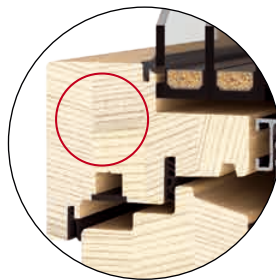
Zafrézovaná zasklívací lišta
